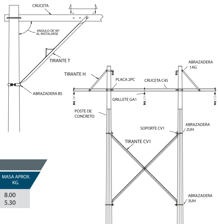
TIRANTE H
