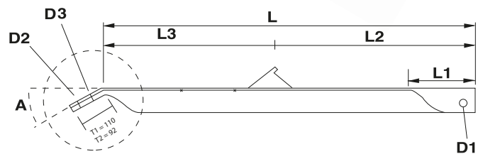
TIRANTE T1, T2
