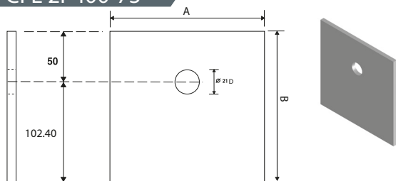
PLACA PL-2 CFE 2P400-73
