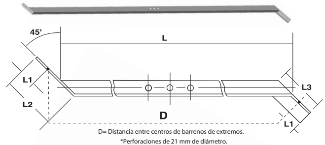
TIRANTE H
