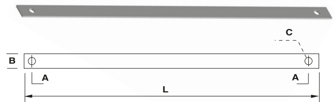
TIRANTE T1, T2
